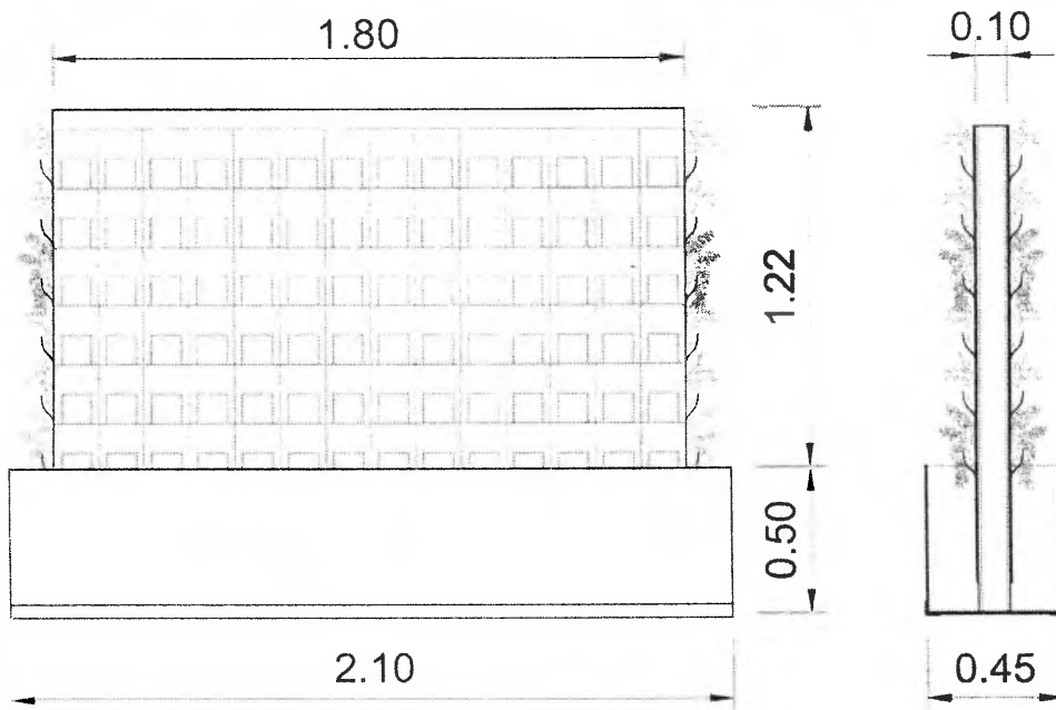
Detalle Tótem Bifaz Móvil con riego automático
